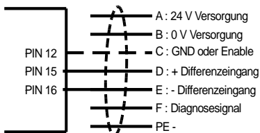
Ventile (6 + PE Stecker) mit integrierter Elektronik, Spannungssignal +/- 10V
