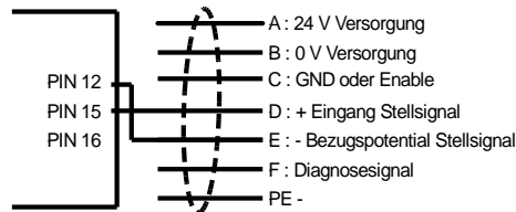
Ventile (6 + PE Stecker) mit integrierter Elektronik Stromsignal 4-12-20 mA
