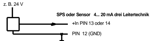
Ventile (6 + PE Stecker) mit integrierter Elektronik Stromsignal 4-12-20 mA
